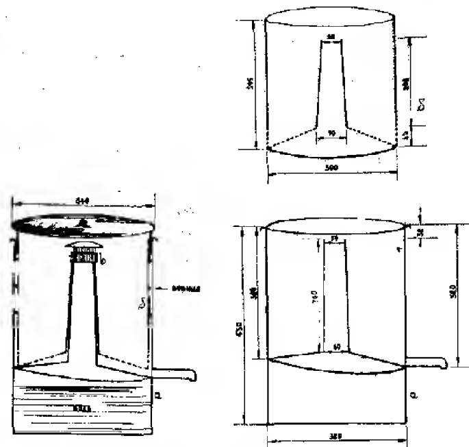
Попречни пресек парног топioniка: два десна казана спојена у један — чине парни топioniк, лево.
